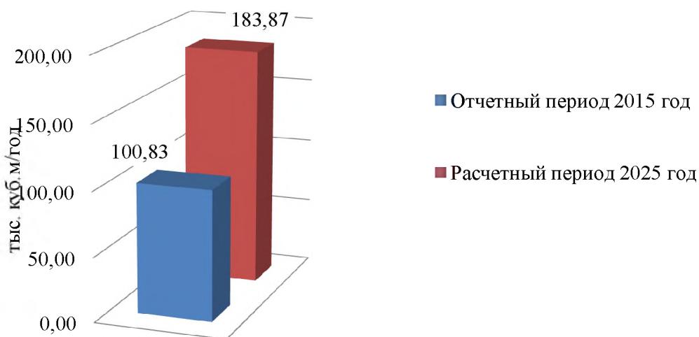
Сравнительная диаграмма существующего и перспективного объема водопотребления пос. Высокогорский
