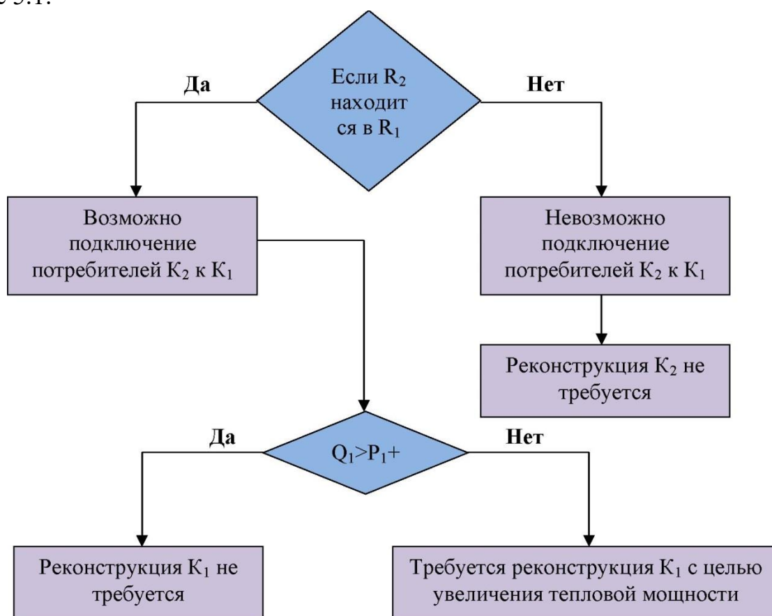
Рисунок 5.1 - Блок-схема обоснования реконструкции котельной K_1 , K_2 - котельная №1 и котельная №2;
