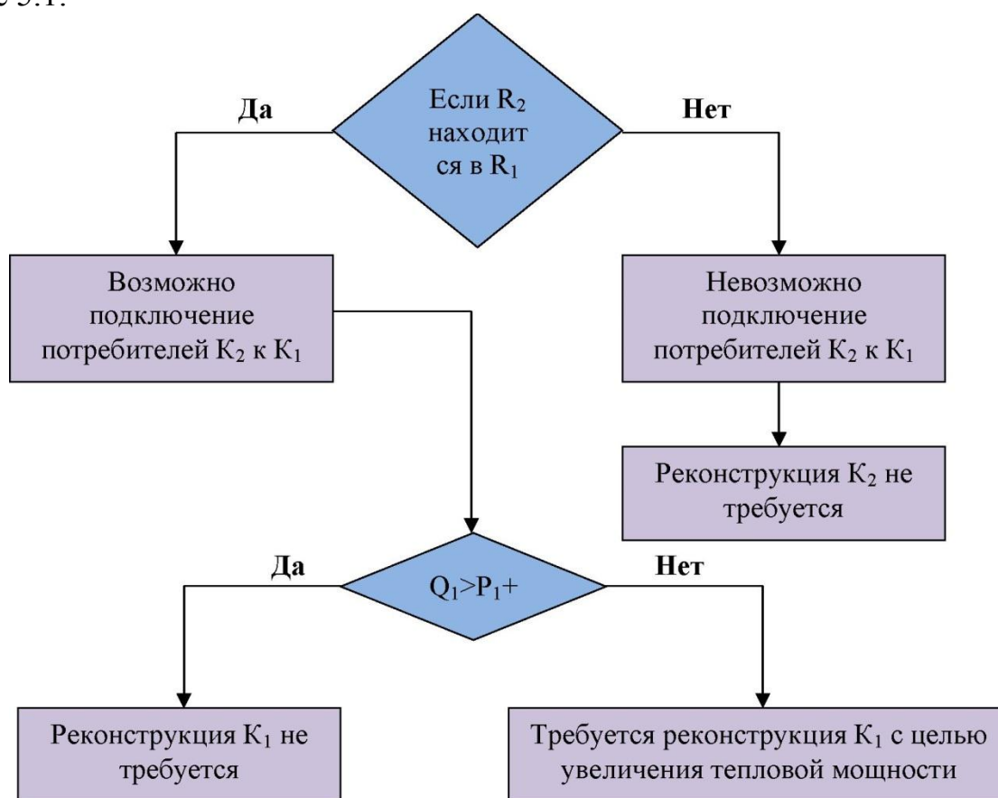
Рисунок 5.1 - Блок-схема обоснования реконструкции котельной K_2 - котельная №1 и котельная №2;
